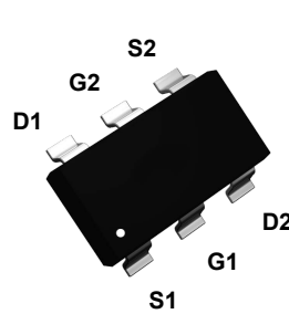
SOT-363
